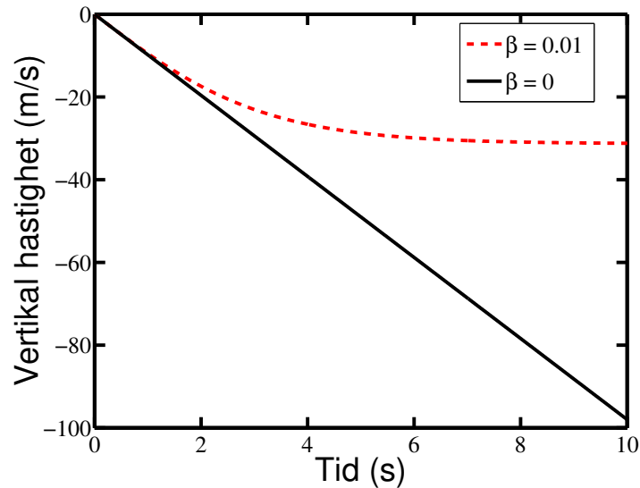
Figur 20: Farten för en fallande kropp utan luftmotstånd ökar linjärt. För \beta = 0.01 är terminalhastigheten ca. 30 m/s, vilket uppnås efter ca. 10 s, se Ekv. (97)
