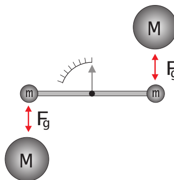
Figur 21: Henry Cavendish mätapparat för att mäta gravitationskonstanten G . Gravitationskraften mellan massiva blykulor och mindre massor får visaren att röra på sig.
