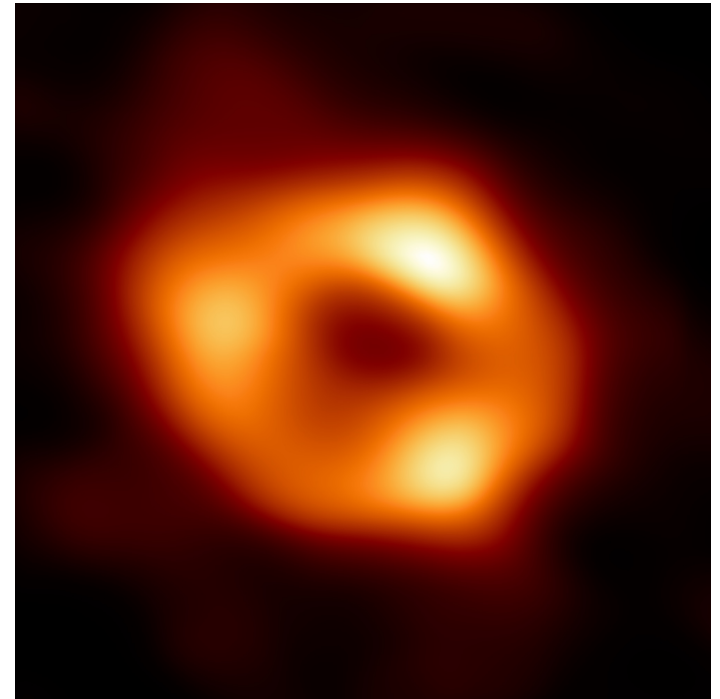
Linnunrata
