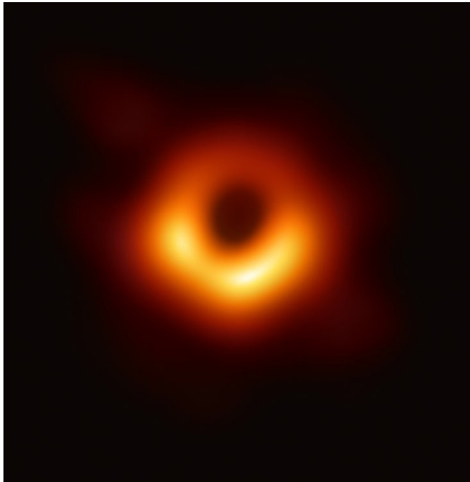
M87
